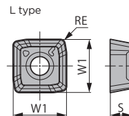
Fig. 3 Centrální destička L type
