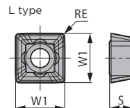
Fig. 1 Obvodová destička L type
