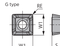
Fig. 2 Obvodová destička G type
